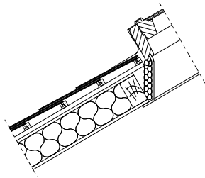
Aansluiting onderaan het dakraam
