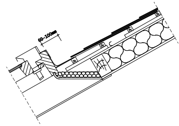
Aansluiting bovenaan het dakraam
